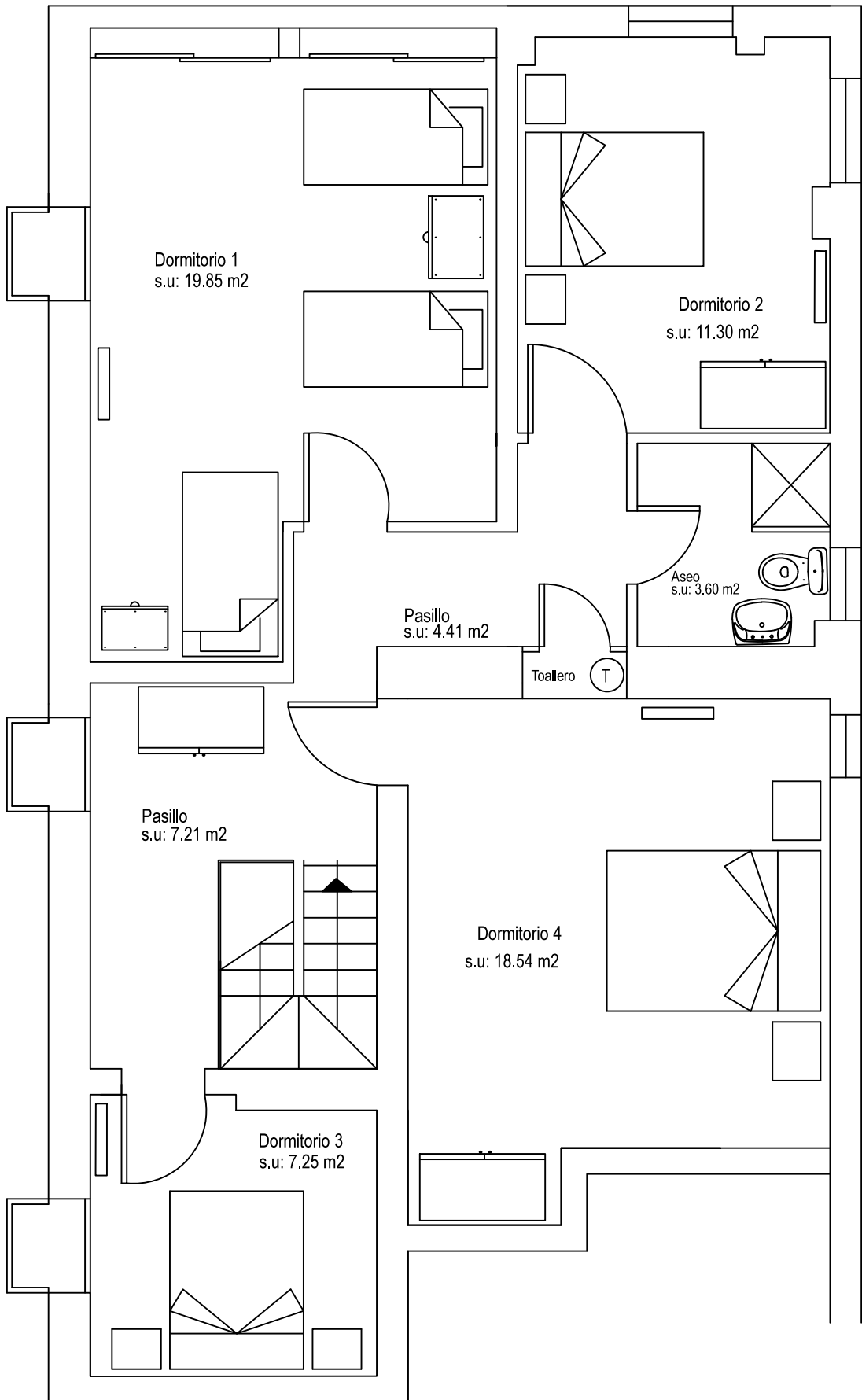
PLANTA PISO
